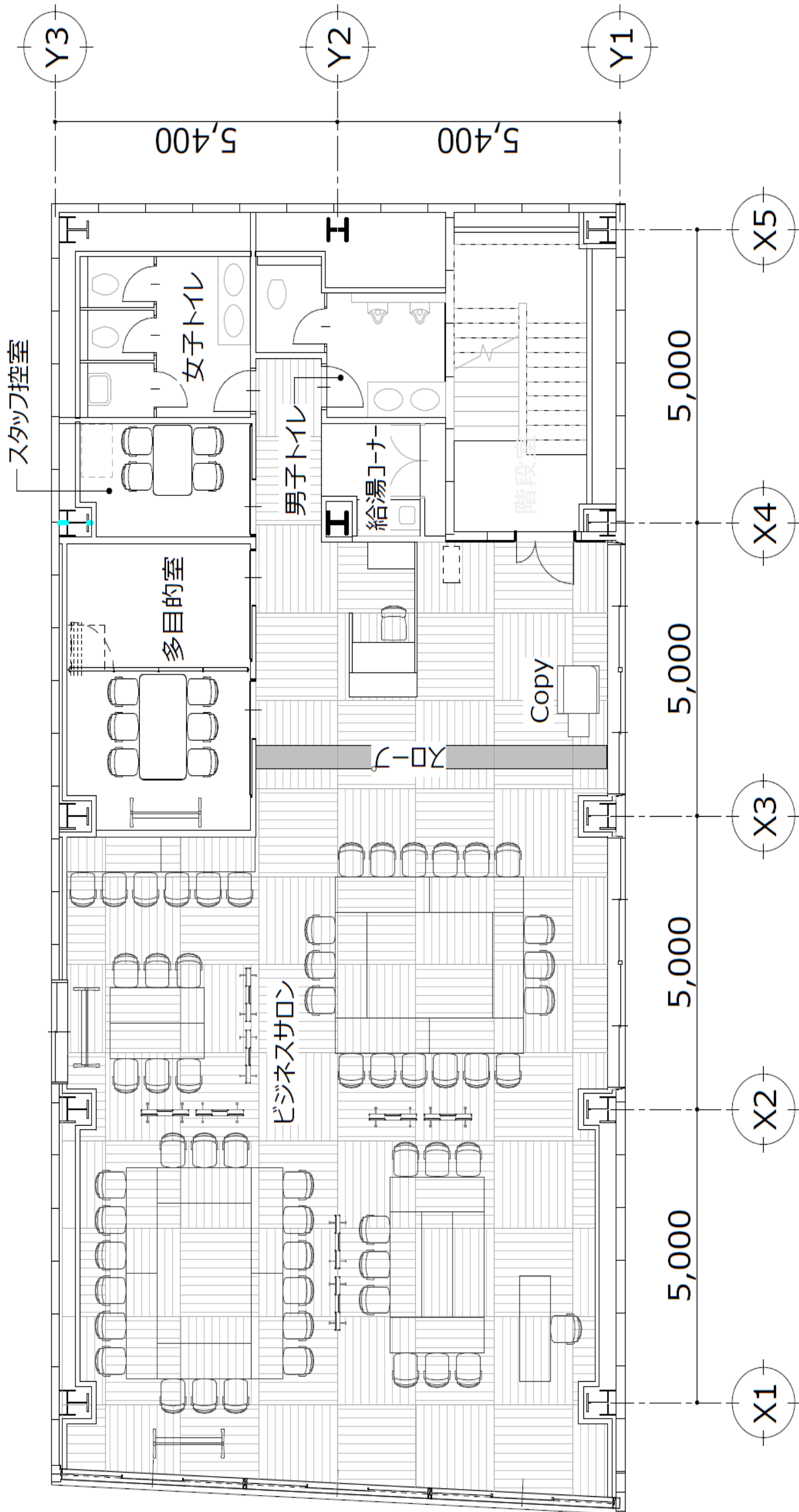
添付資料a.2Fフロア利用平面図
